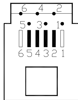
Схема эл.принципиальная элемента сетевого обрамления iB-Vox-Clip
