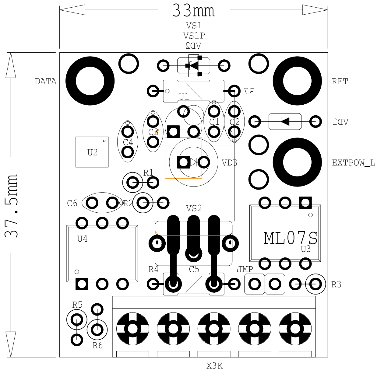
Схема размещения компонентов на плате ML07S, используемой для построения устройства ML-OEM типа ML07S
